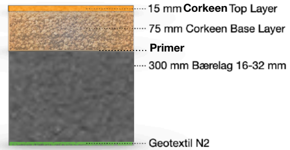
Fallhøyde 2,3 m
